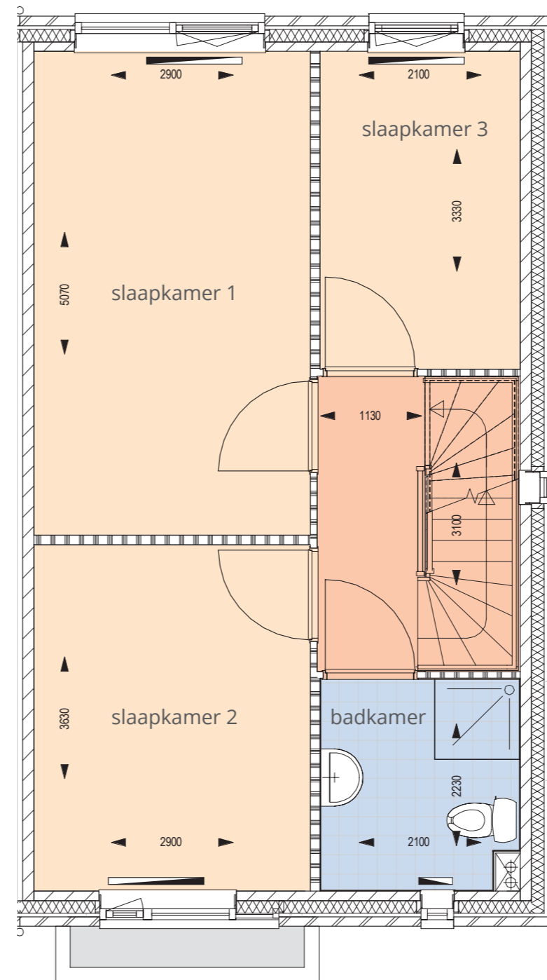
1 e verdieping
