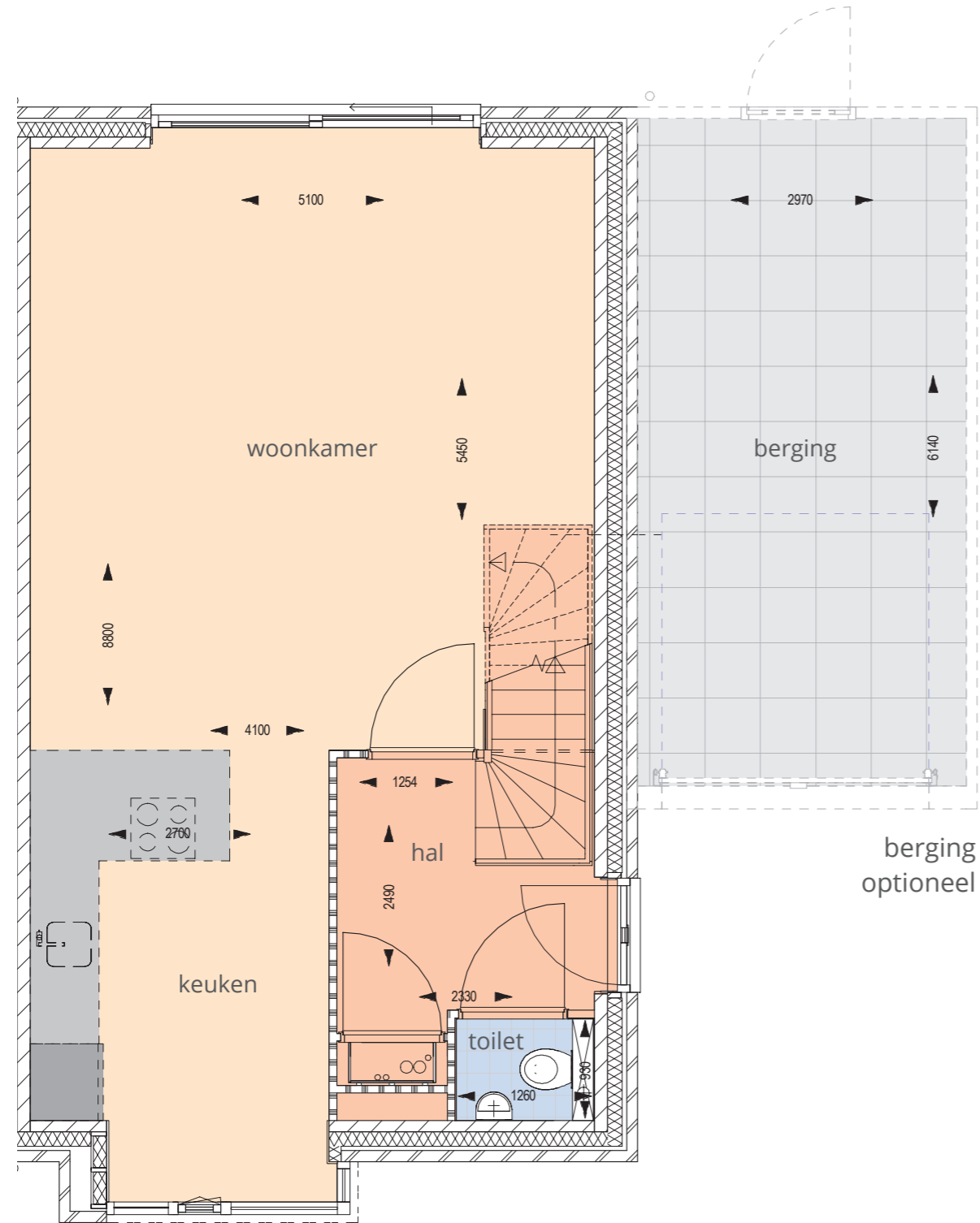
begane grond
