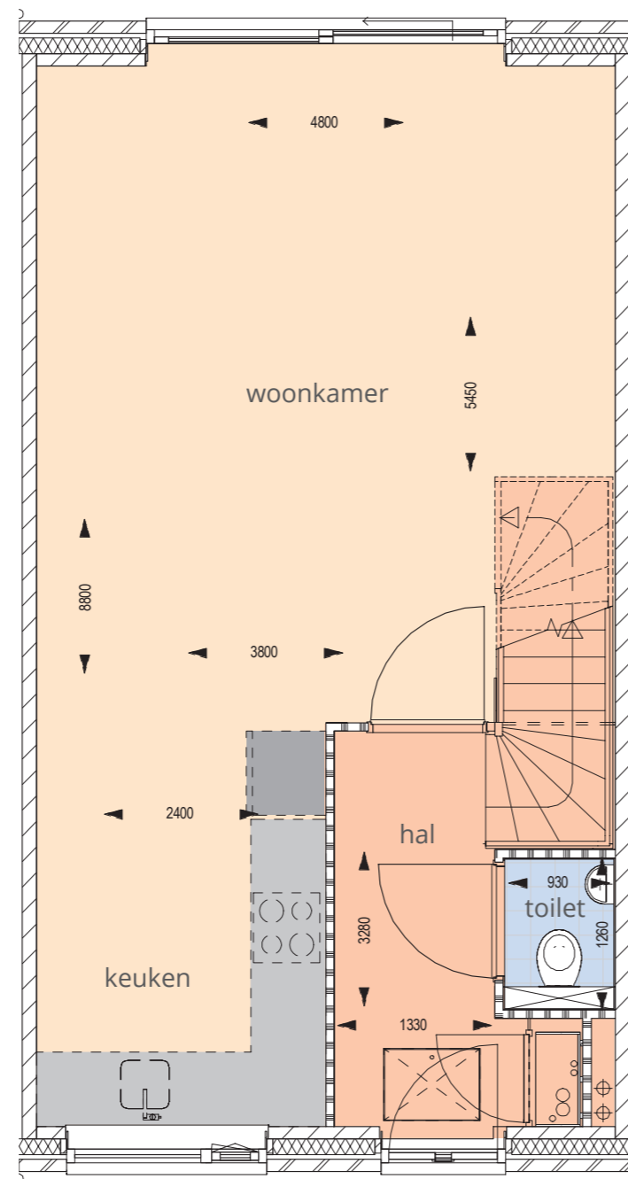
begane grond
